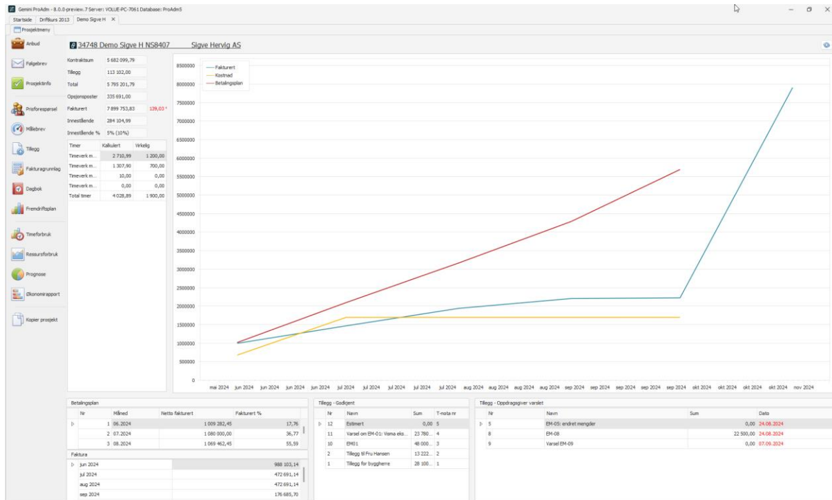
Figur 8: Prosjektmeny grafer
